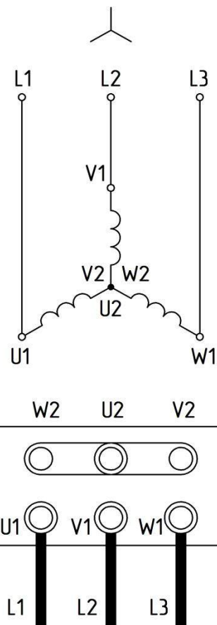
Схема соединения звезда
